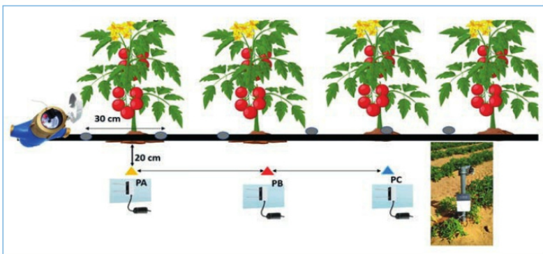
FIG. 3 Esquema de la instalación de los sensores en el campo.
