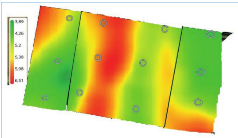
FIG. 2 Mapa de conductividad eléctrica aparente del suelo (mS/m) a 0-0,5 m.
